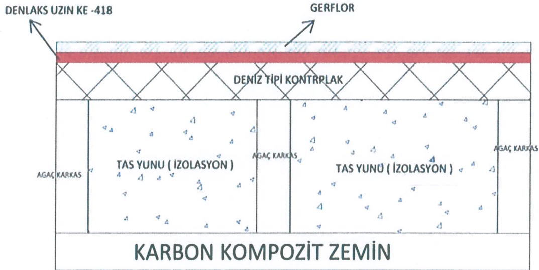
Şekil 3.1. Zemin üstü izolasyon ve kaplama tabakalarını gösterir resim
